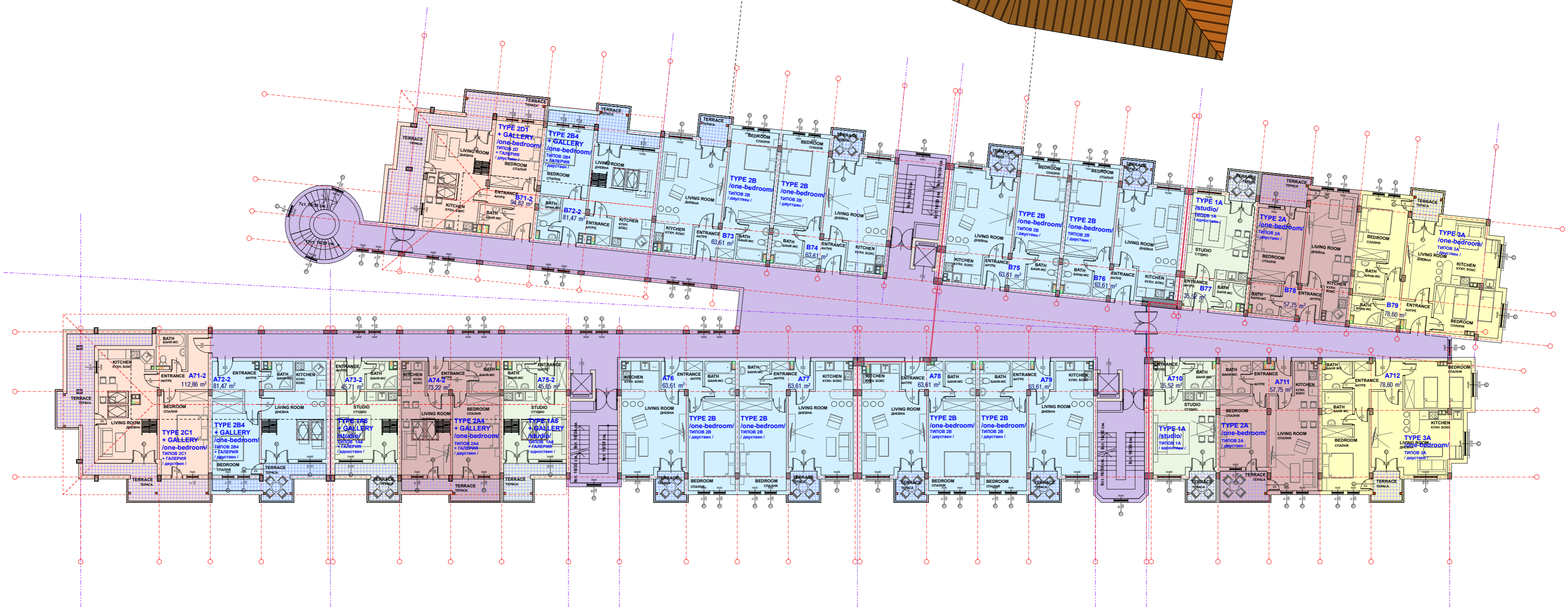
PLAN 7th STORY LEVEL +20,80 scale 1'200 РАЗПРЕДЕЛЕНИЕ СЕДМИ ЕТАЖ КОТА +20,80 М 1'200
