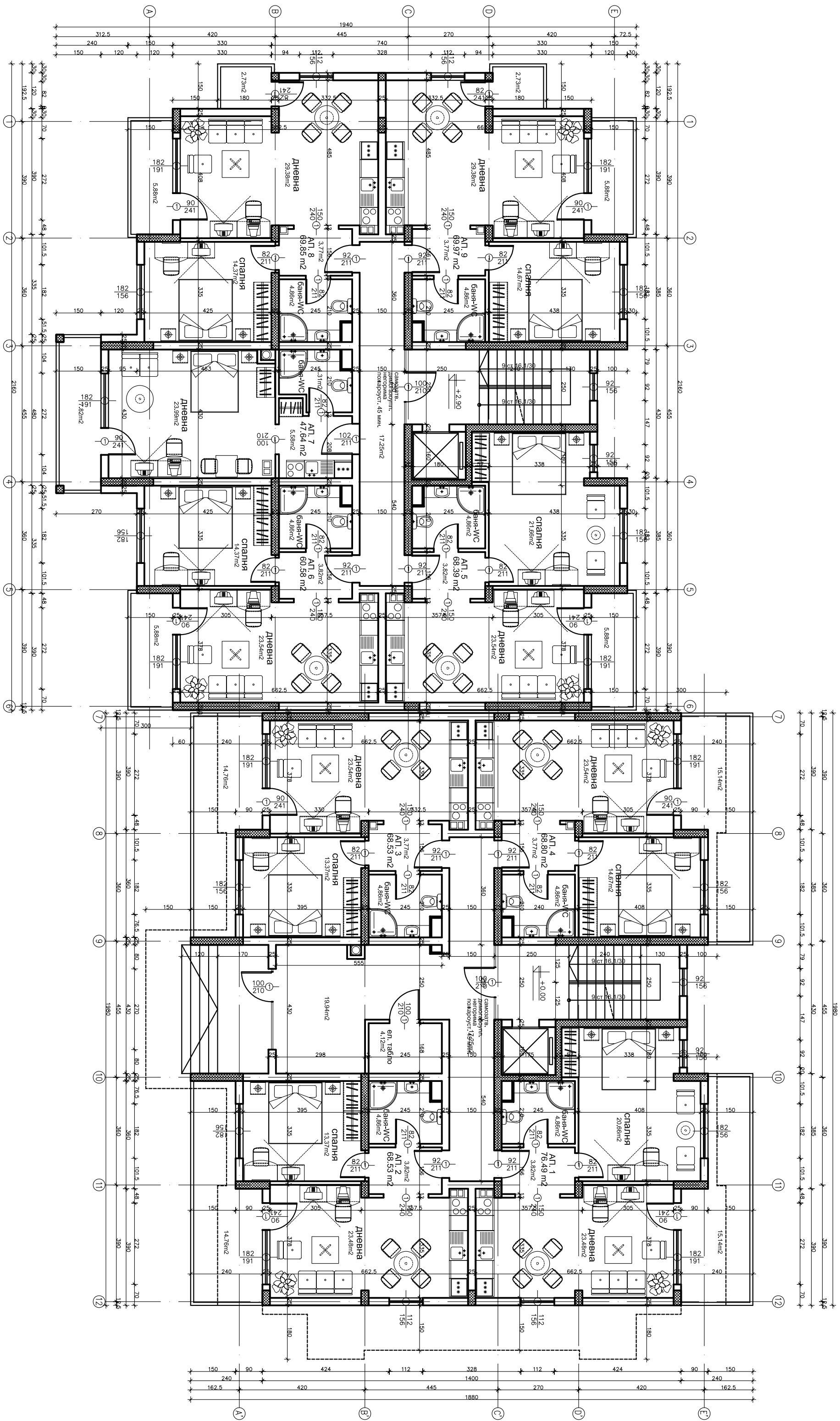
РАЗПРЕДЕЛЕНИЕ КОТА +2.90
