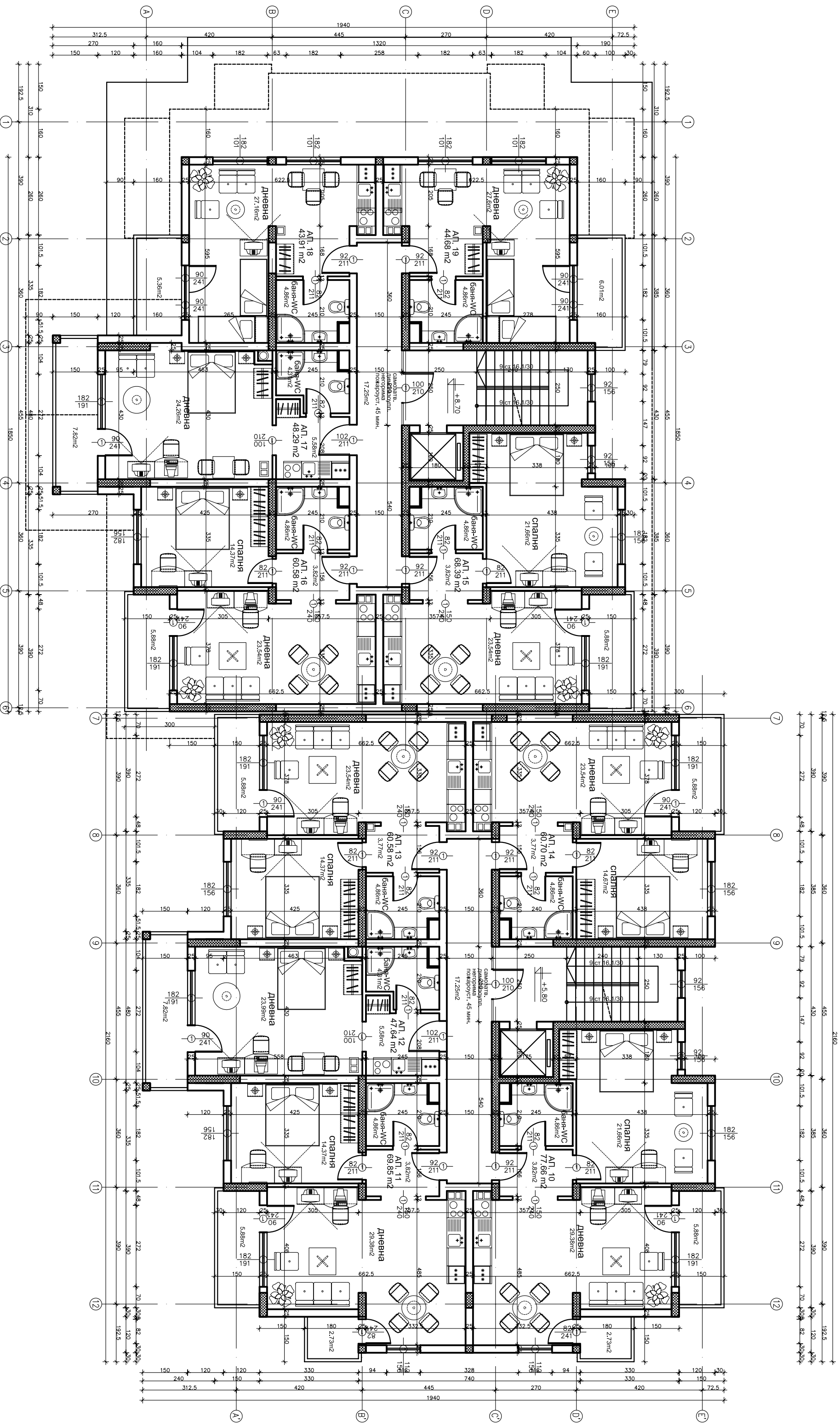
РАЗПРЕДЕЛЕНИЕ КОТА +8.70
