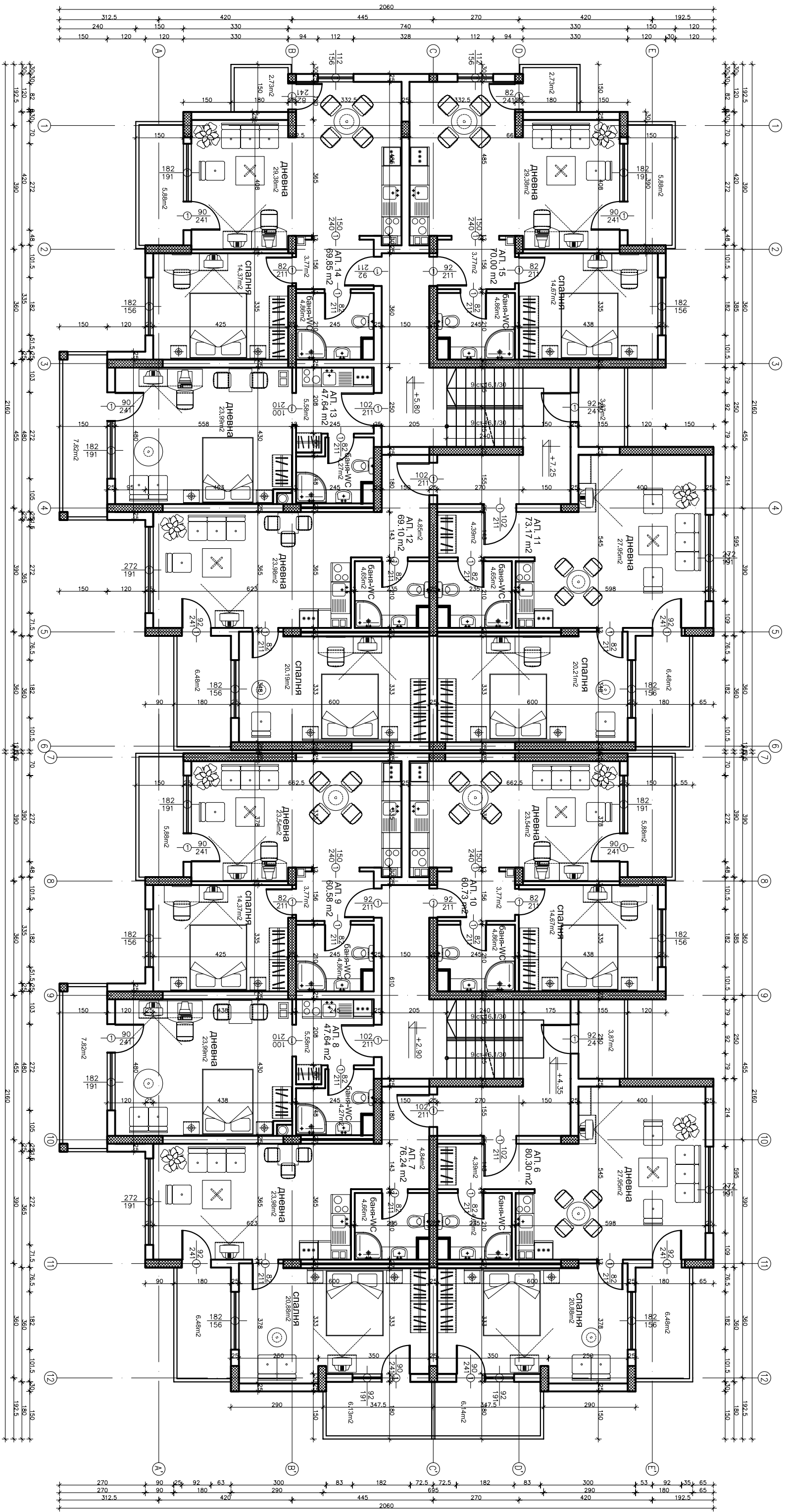
РАСПРЕДЕЛЕНИЕ КОТА +5.80
